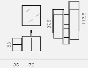
E.GÒ nodo step 36 (page 38-39) L 105 x P 51 cm + pensili / wall units
